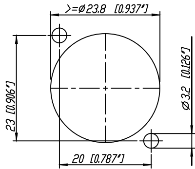
Frontplattenausschnitt (Frontseite) Panel cut out (front side)
