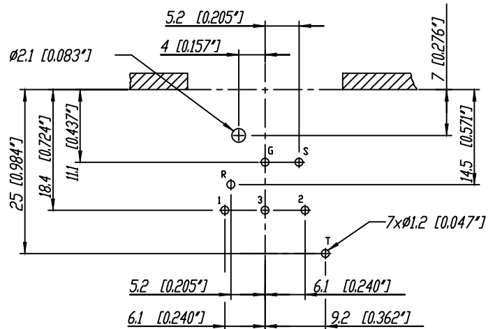
Print-Bohrplan (Bestueckungsseite) PCB-Layout (component side)
