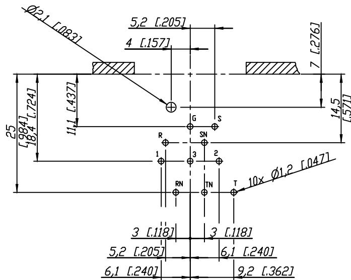
Print-Bohrplan (Bestueckungsseite) PCB-Layout (component side)
