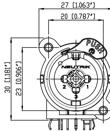
Frontplattenausschnitt (Frontseite) Panel cut out (front side)
