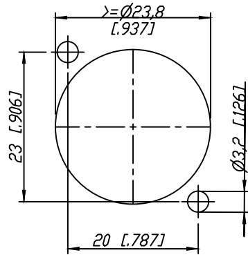
Frontplattenausschnitt (Frontseite) Panel cut out (front side)
