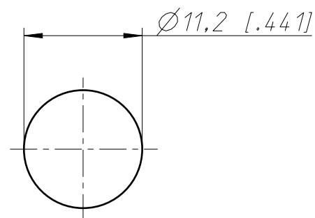
Frontplattenausschnitt (Rückseite) Panel cut out (rear side)
